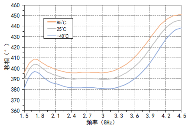
移相VS频率@Vt=14V
