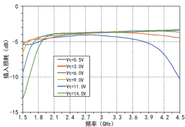
插入损耗VS频率@Pin=-10dBm
